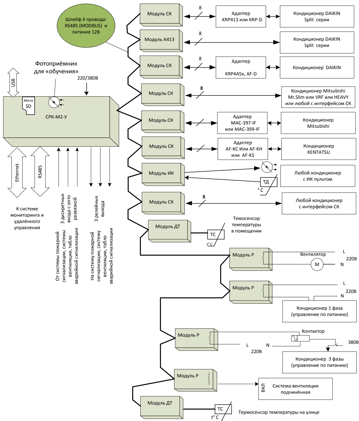
Рисунок 1- Структурная схема системы на базе СРК-M2
